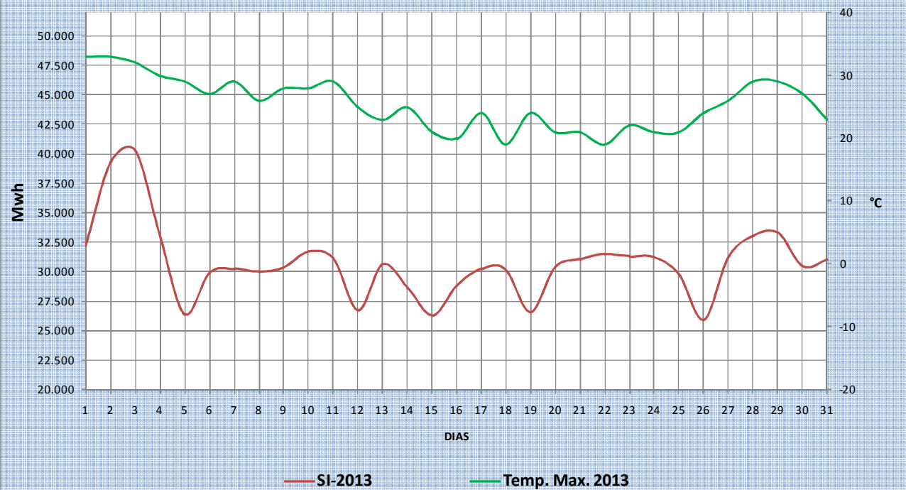
DEMANDA DE ENERGIA SISTEMA INTERCONECTADO (SI) - MAYO / 13
