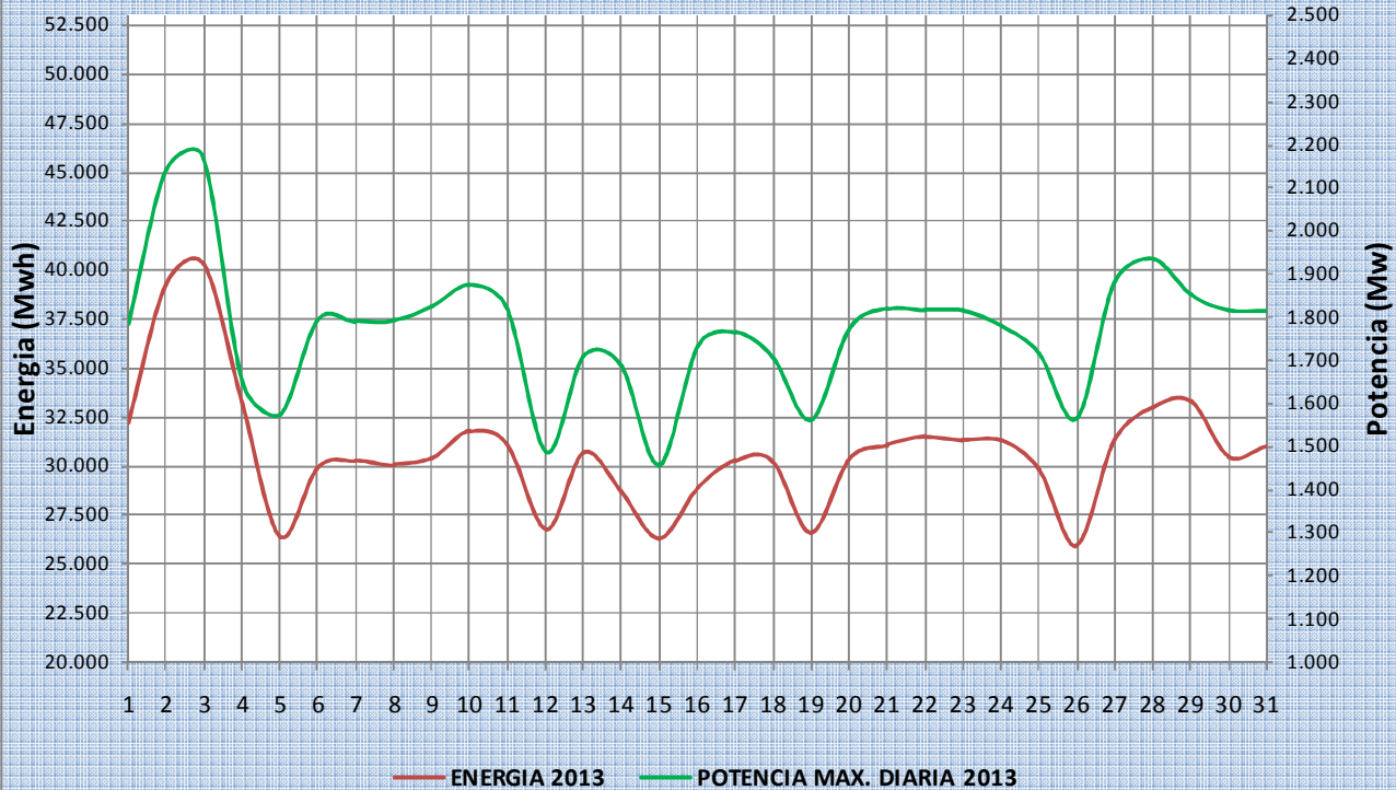
DEMANDA DE ENERGIA Y POTENCIA MAXIMA DIARIA SISTEMA INTERCONECTADO (SI) MES : MAYO / 13
